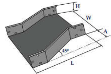
Co Z ngang phải Right horizontal Z
