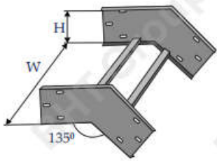
Co xuống 45° External riser 45°
