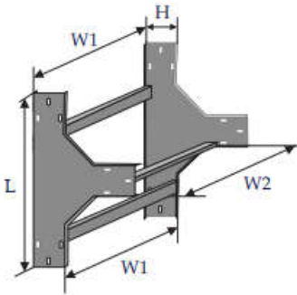
Co T đứng trục dọc T shaped hinge vertical
