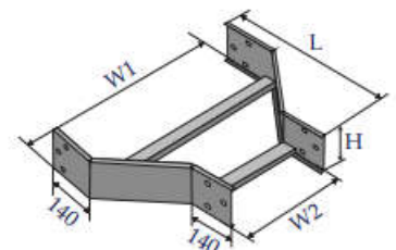
Co giảm giữa Offset reducer
