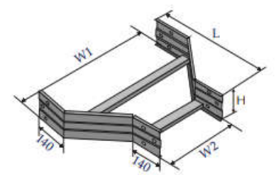
Co giảm giữa Offset reducer
