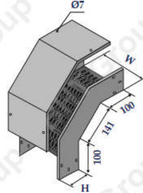
Co xuống 90° External riser 90°
