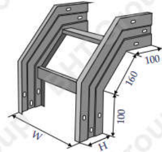
Co xuống 90° External riser 90°
