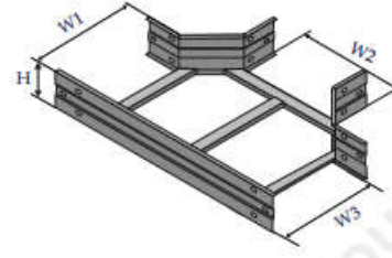
Co chữ T Horizontal T
