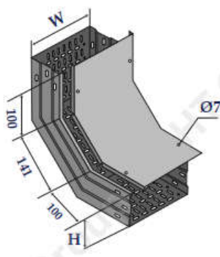
Co lên 90° Internal riser 90°
