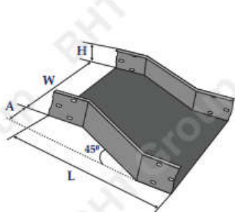
Co Z ngang trái Left horizontal Z
