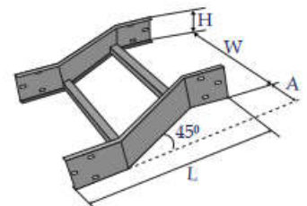
Co Z ngang phải Right horizontal Z
