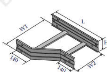
Co giảm phải Right reducer
