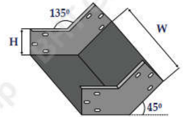
Co lên 45° Internal riser 45°
