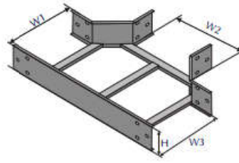
Co chữ T Horizontal T
