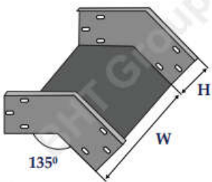
Co xuống 45° External riser 45°
