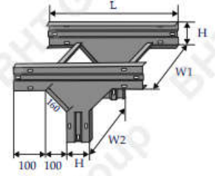
Co T đứng trực ngang T shaped hinge horizontal
