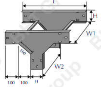
Co T đứng trục ngang T shaped hinge horizontal
