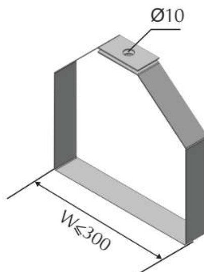
Cùm Treo Máng Cáp Clevis hange
