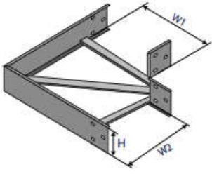
Co ngang 90° Horizontal elbow 90°
