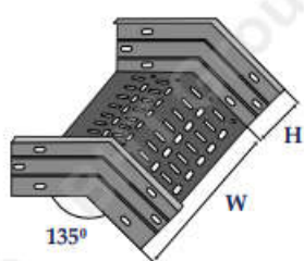
Co xuống 45° External riser 45°
