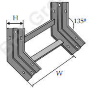
Co lên 45° Internal riser 45°
