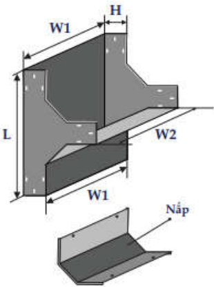
Co T đứng trục dọc T shaped hinge vertical
