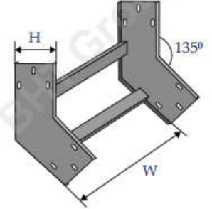
Co lên 45° Internal riser 45°
