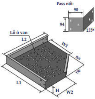
Co ngang 90° Horizontal elbow 90°
