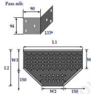
Co chữ T Horizontal T
